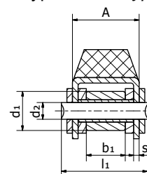
Typ 2V / 2V Type
