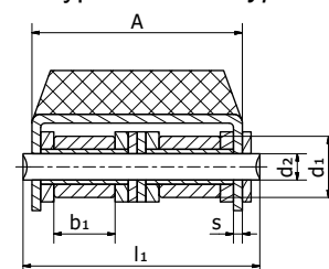
Typ G-2 / G-2 Type
