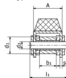
Typ G-2 / G-2 Type
