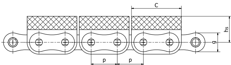
Typ G-1 / G-1 Type Typ G-2 / G-2 Type
