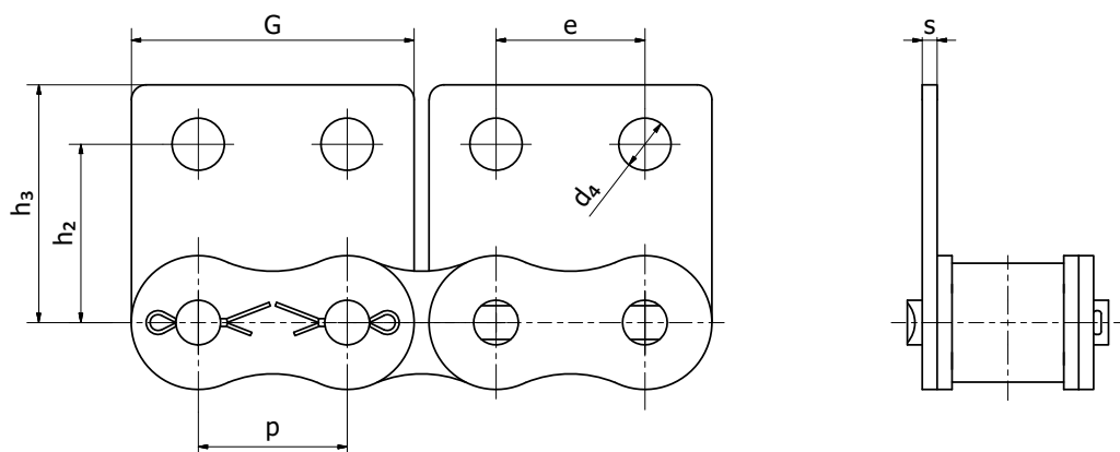
M7: Hranatý unašeč rovný, 2 díry, 1 strana / M7: Square attachment - straight, 2 holes, 1 side
