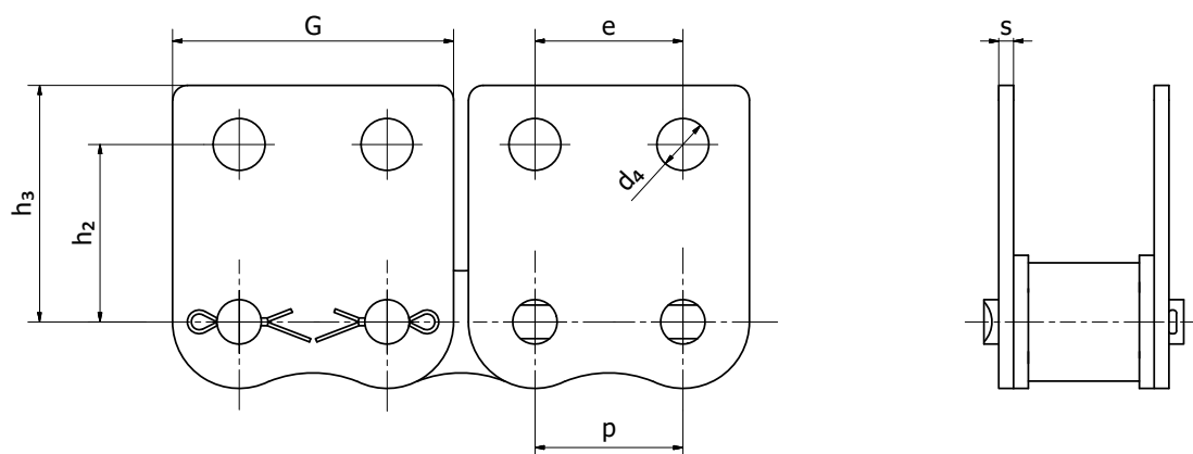
M8: Hranatý unašeč rovný, 2 díry, 2 strany / M8: Square attachment - straight, 2 holes, 2 sides
