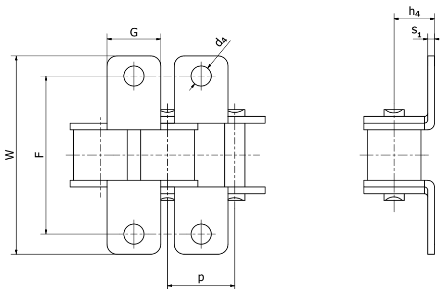
K2: Hranatý unašeč 90°, 1 díra, 2 strany / K2: Square attachment 90°, 1 hole, 2 sides
