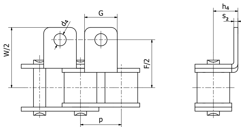
K1: Hranatý unašeč 90°, 1 díra, 1 strana / K1: Square attachment 90°, 1 hole, 1 side
